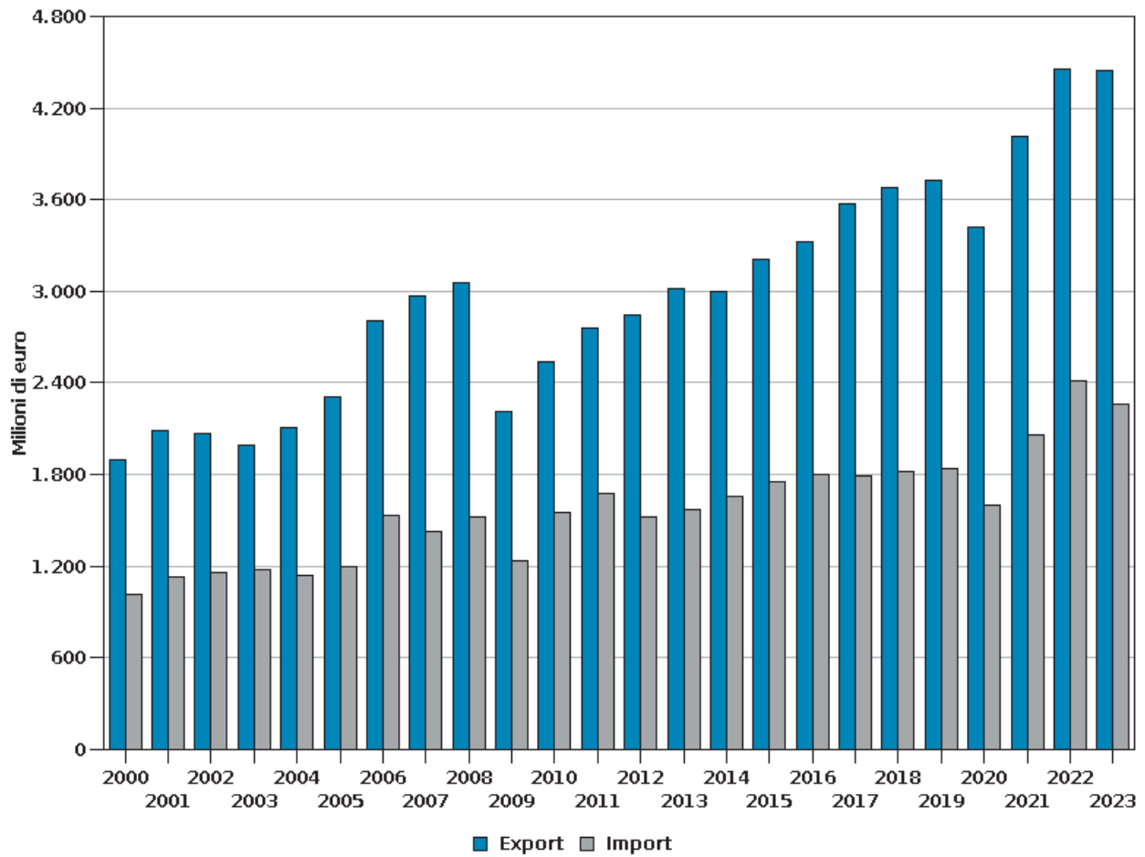
FIG. CE.06 - Import ed export - Serie storica della provincia di Forlì-Cesena
